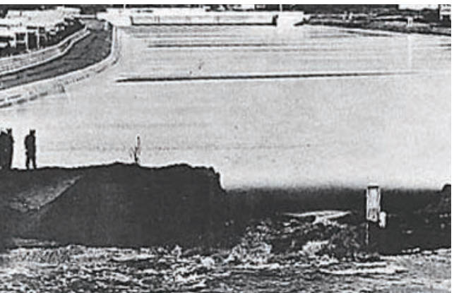
茨戸川の洪水を直接日本海に流す石狩放水路 「一般財団法人 石狩川振興財団 HP より」
