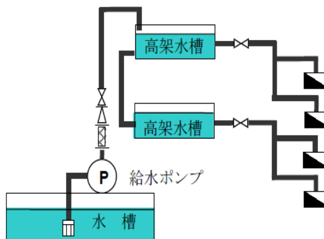
第2-5図 高架水槽の設置高さを考慮して設ける方法の例
