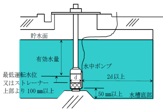
第 2-11 図 水中ポンプを設ける場合
