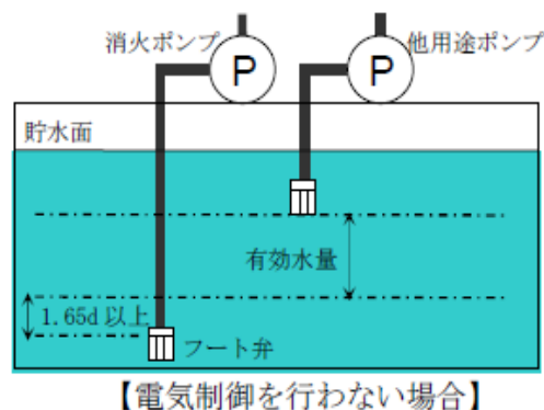
第 2-13 図 地下又は床下水槽の場合
