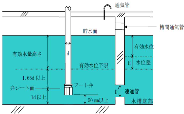
第 2-10 図 複数の水槽を連通管により接続して使用する場合
