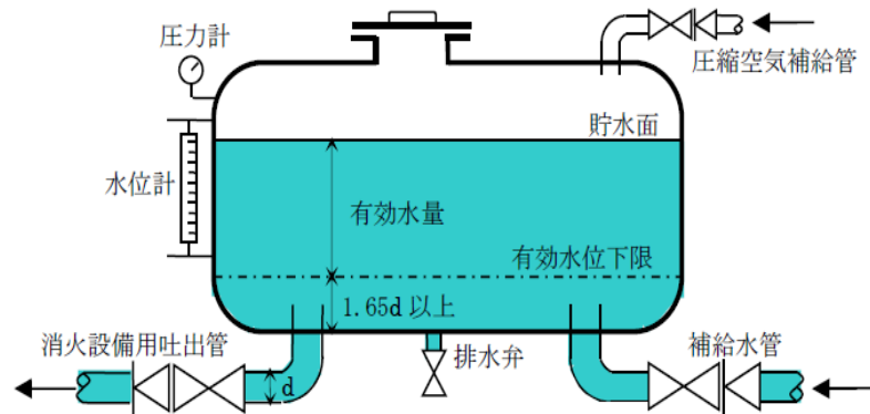
第 2-14 図 圧力水槽の場合
