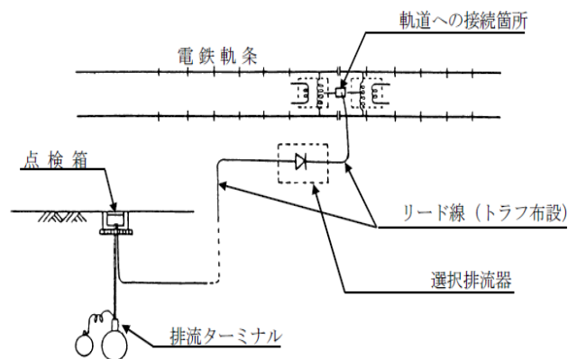
第 2-17 図 選択排流方式の施工例
