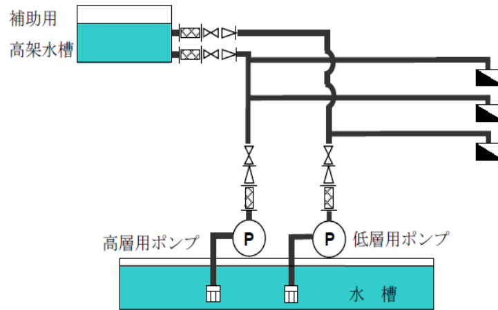
第 2-6 図 ポンプ揚程を考慮し配管を別系統にする方法の例
