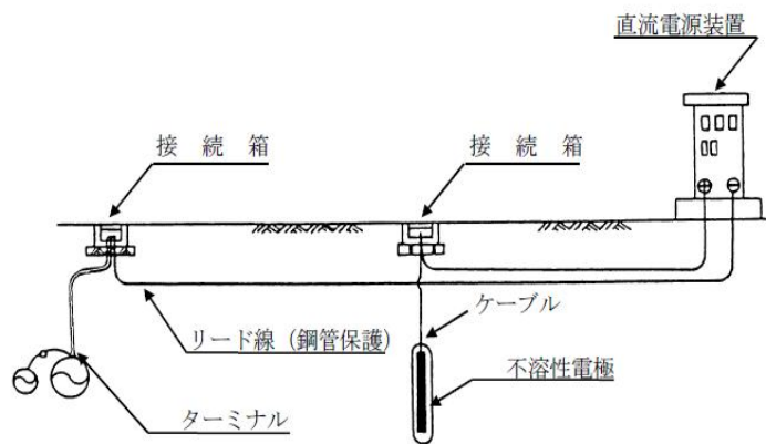
第 2-16 図 外部電源方式の施工例
