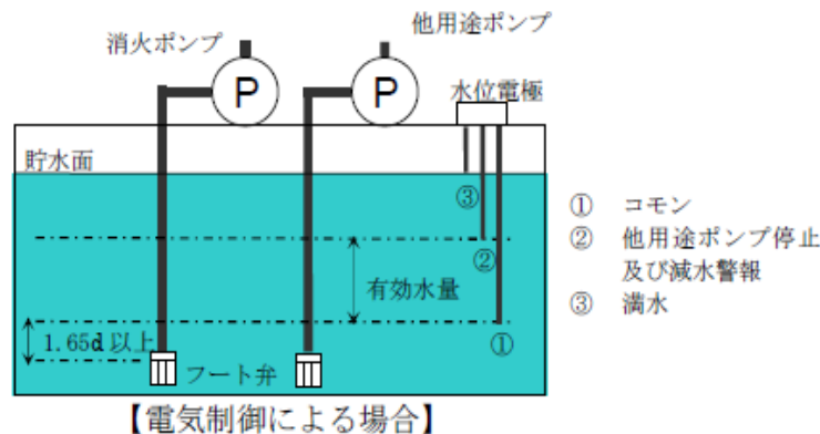
第 2-12 図 地上又は床上水槽、高架水槽の場合 (イ) 地下又は床下水槽 (第 2-13 図参照)
