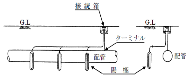
第 2-15 図 放電陽極方式の施工例
