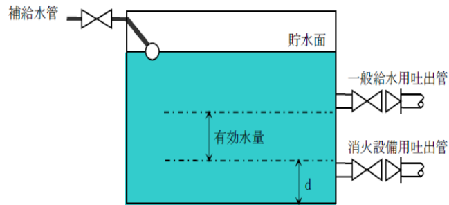
第 2-12 図 地上又は床上水槽、高架水槽の場合 (イ) 地下又は床下水槽 (第 2-13 図参照)
