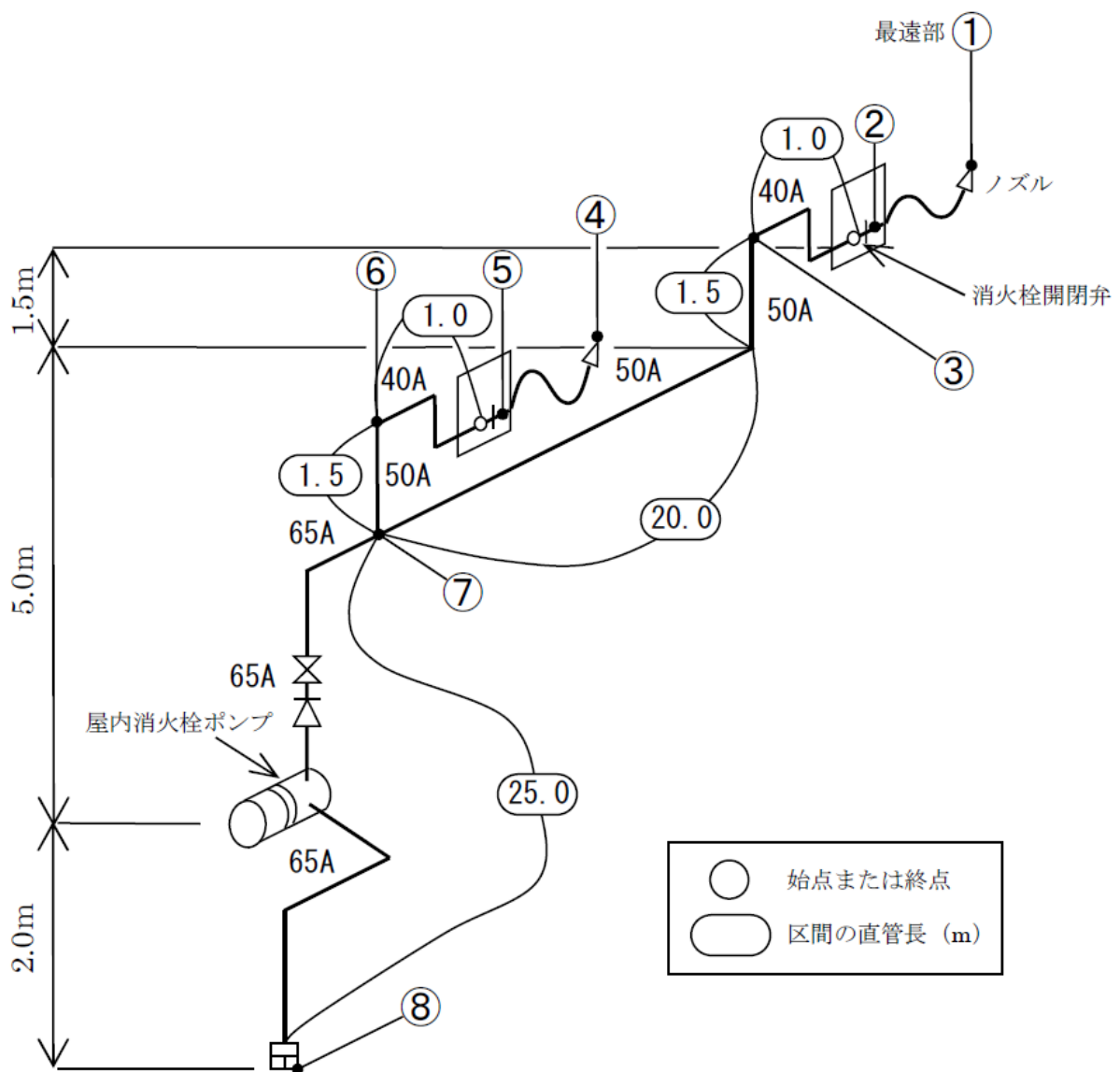
図 1 号消火栓の摩擦損失計算図
